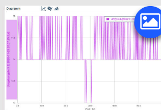
Освещенность
