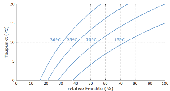
Kuva 7 : Kastepiste 4 eri lämpötilassa
